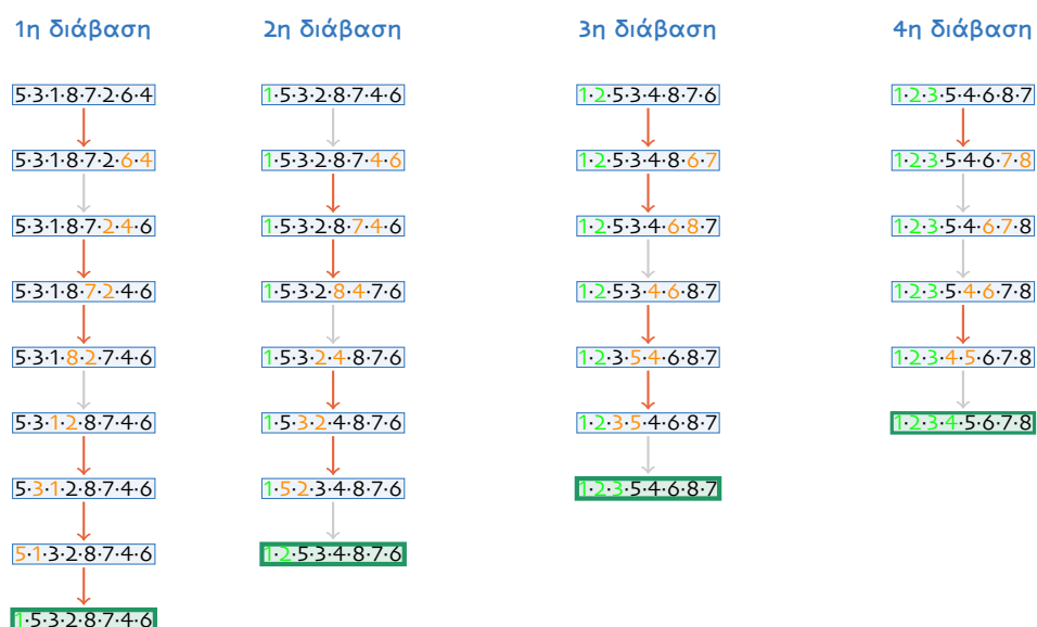
Σχήμα 5.14: Bubble Sort
