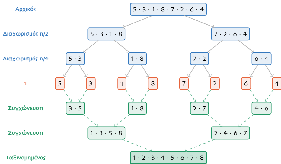
Σχήμα 5.15: Merge Sort
